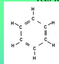
Benzene molecule
