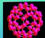
C-60 molecule
