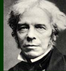
M. Faraday (1791-1867)
